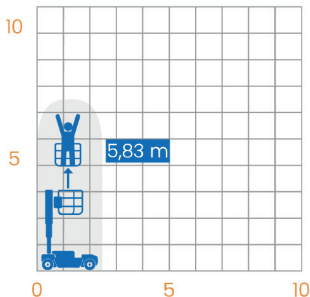
SNORKEL 1230 E
